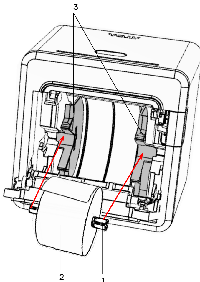
Рисунок 16. Заправка бумаги при вертикальной установке ККТ
