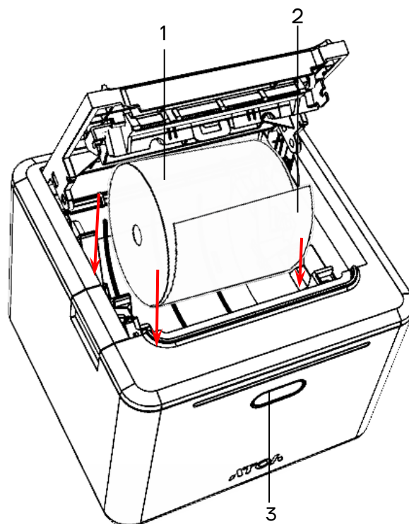
Рисунок 12. Заправка бумаги при горизонтальной установке ККТ
