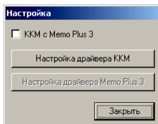
Рисунок 34. Окно Настройка
